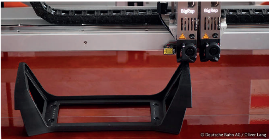
»Mobility goes Additive« Projekt der Deutschen Bahn, 3D-Druck einer Kopfstütze für einen Regionalzug
