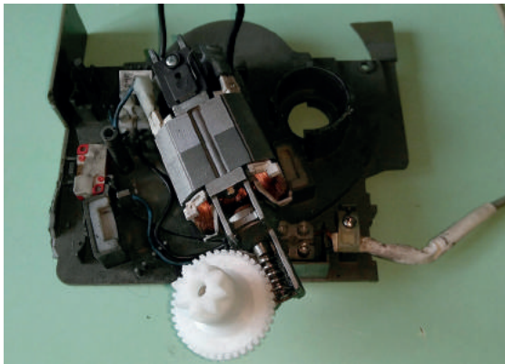
oben abgenutztes Motorzahnrad links 3D-reparierter Motorblock
